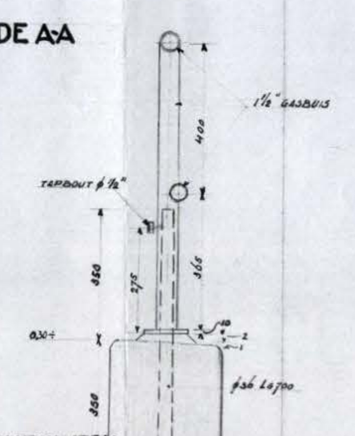
DSN.OVER HEKWERK
