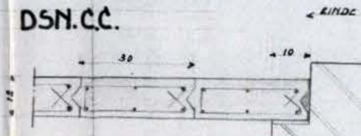
AANSLUITING DAM-WAND AAN VLEUGEL
